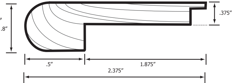
Flushmount Stairnose- EGD 1/2"
