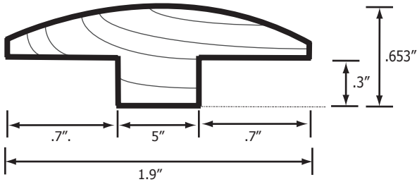
T-Mold
