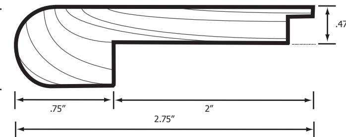
Flushmount Stairnose- EGD 1/2"
